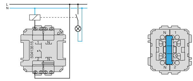
Kuva 6: Valaistu kuorman ollessa poiskytkettynä (hakuvalo), painike sulkeutuvalla koskettimella ja merkintäikkunalla esim. turvasovellukset. LED-elementti kytketty välille 2 - 1.
