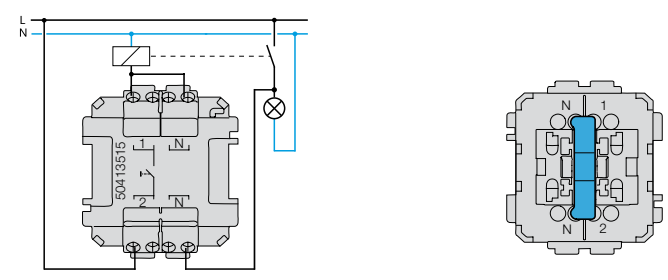
Kuva 7: Valaistu kun kuorma päällä (kontrollikytkin), painike sulkeutuvalla koskettimella ja merkintäikkunalla esim. valaistavien ulkoalueiden ohjaukseen. LED-elementti kytketty välille N - N.
