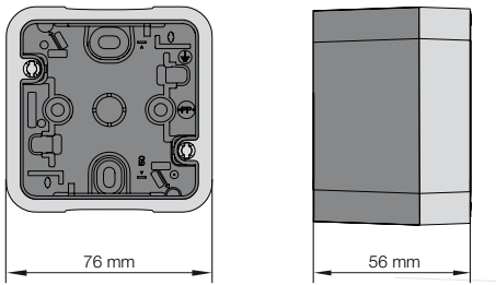
Kuva 16: Kotelo pinta-asennettava
