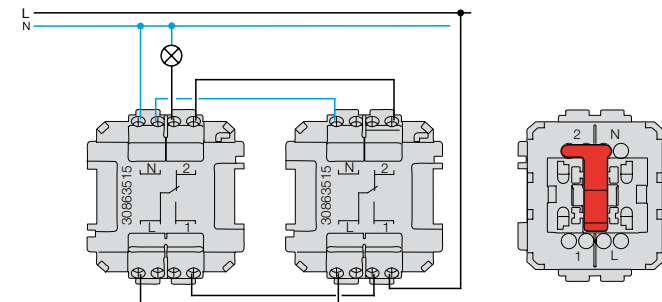
Kuva 4: Valaistu kun kuorma päällä (kontrollikytkin), porraskytkeä 2:lla linssillisellä vaihtokytkimellä. LED-elementti kytketty välille 2 - N.
