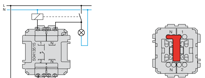
Kuva 8: Valaistu kun kuorma päällä (kontrollikytkin), painike sulkeutuvalla koskettimella ja merkintäikkunalla esim. valaistavien ulkoalueiden ohjaukseen. LED-elementti kytketty välille N - 1.
