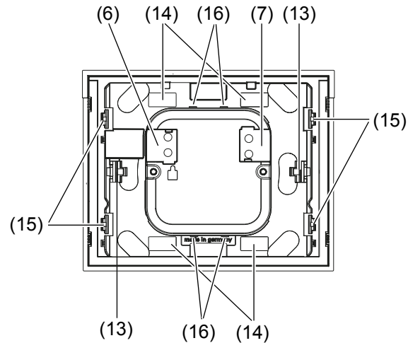
Figura 11: vista posteriore
