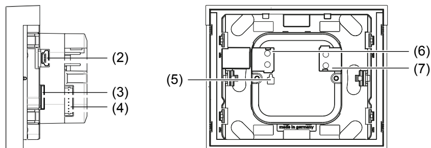
Afb. 2: zij-/achteraanzicht
