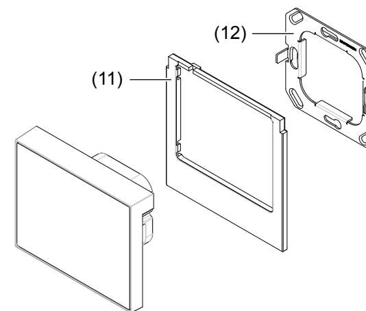
Afb. 10: montage
