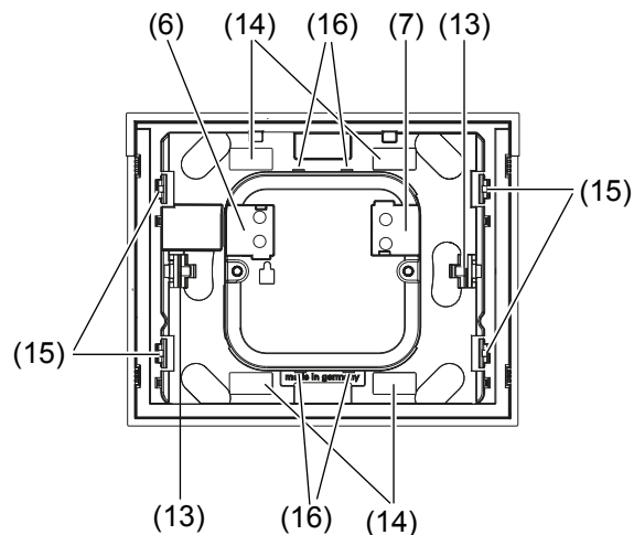
Afb. 11: achteraanzicht
