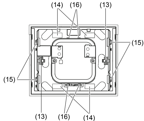
Bild 11: Rückansicht
