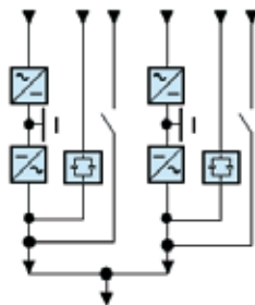
Reduntanttinen modulaarinen UPS (N+1)
