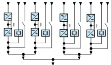
Reduntanttinen UPS-järjestelmä (2N)
