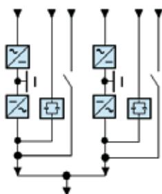
Reduntanttinen modulaarinen UPS (N+1)
