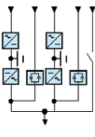
Reduntanttinen UPS-laitos (N+1)
