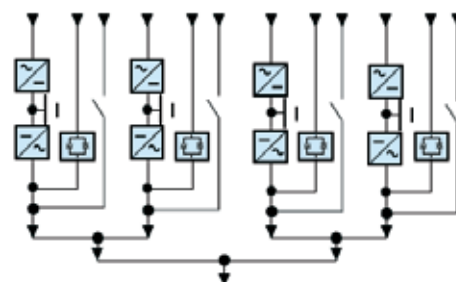
Reduntanttinen UPS-järjestelmä (2N)
